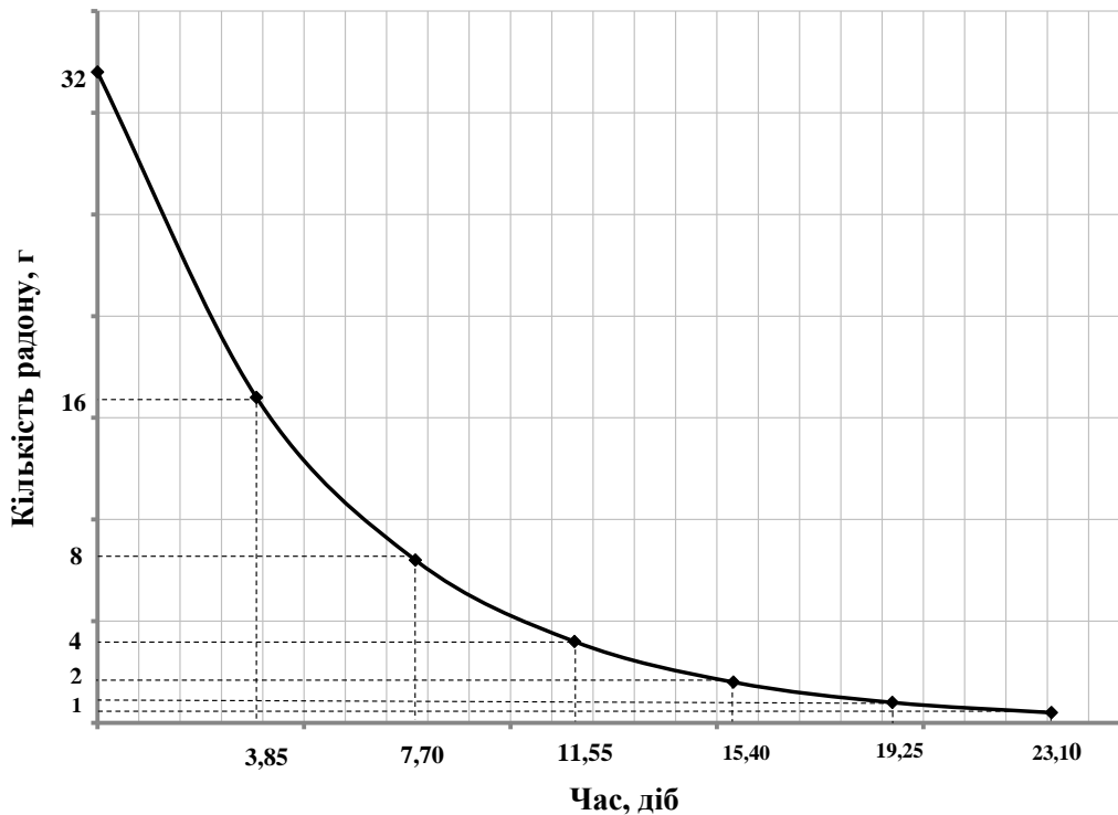
Рис. 1. Швидкість розпаду радону
