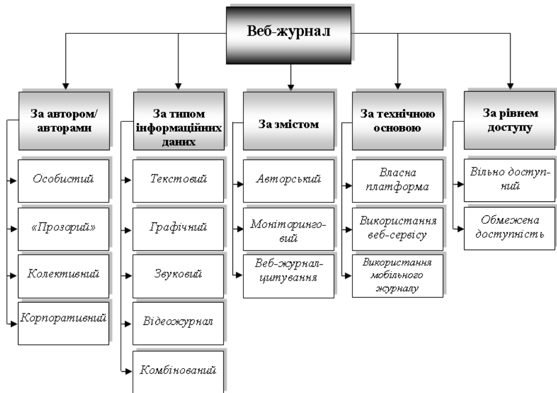
Рис.1.7. Класифікація веб-журналів
