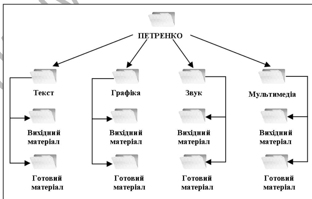
Рис.2.1. Структура папок
