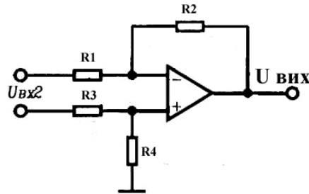
Рис. 3 Електрична схема вимірювального каналу приладу індукційного типу на операційних підсилювачах для вимірювання обертового моменту
