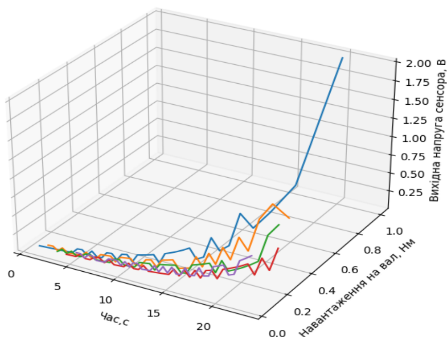
Рис. 6 Результат моделювання вимірювальної системи на базі індуктивних сенсорів.
