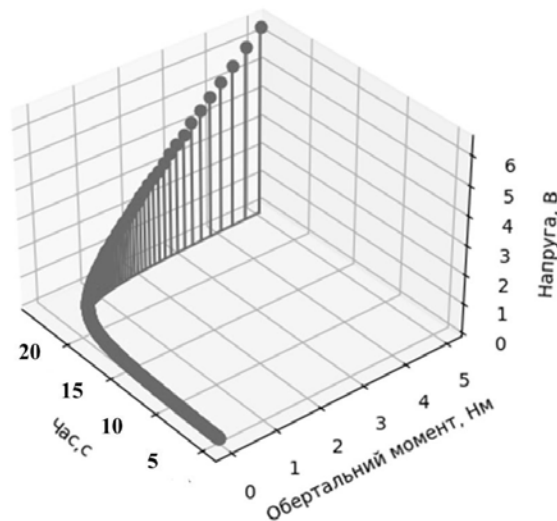
Рис. 3 Часові характеристики залежності обертового моменту та вихідної напруги.
