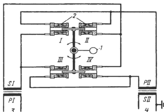
Рис. 2 Схема роботи індуктивного перетворювача обертального моменту, [4]
