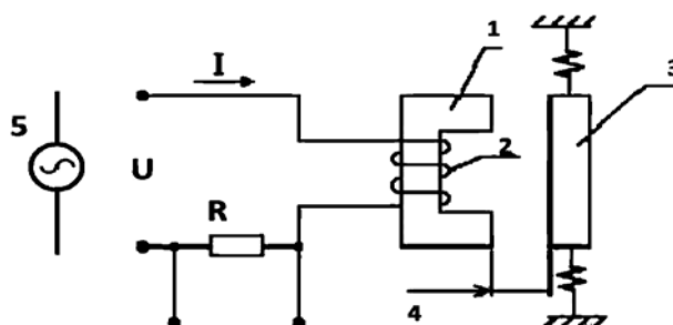
Рис.1 Підключення індуктивного датчика
