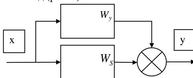
Рис. 5 Структурна схема передатної функції індуктивного сенсора
