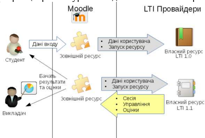
Рис. 1. Архітектура додатку
