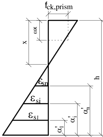
Рис. 7. Схема до розрахунку за інженерною методикою
